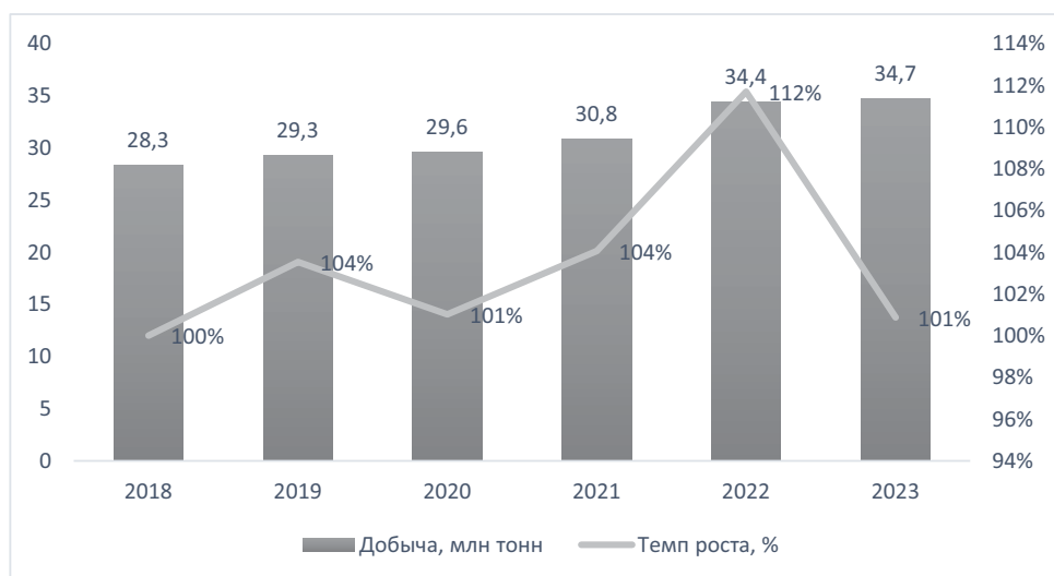
Рис. 3. Динамика добычи газового конденсата в России, млн т 1
