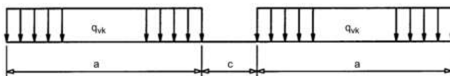
شکل پ-۷- مدل‌های بارگذاری SW/0 و SW/2 [50]
