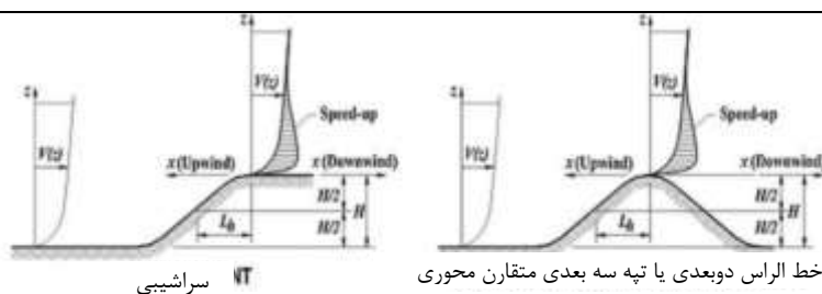
خط الراس دوبعدی یا تپه سه بعدی متقارن محوری ضرایب عارضه‌نگاری برای رده C ۲،۱
