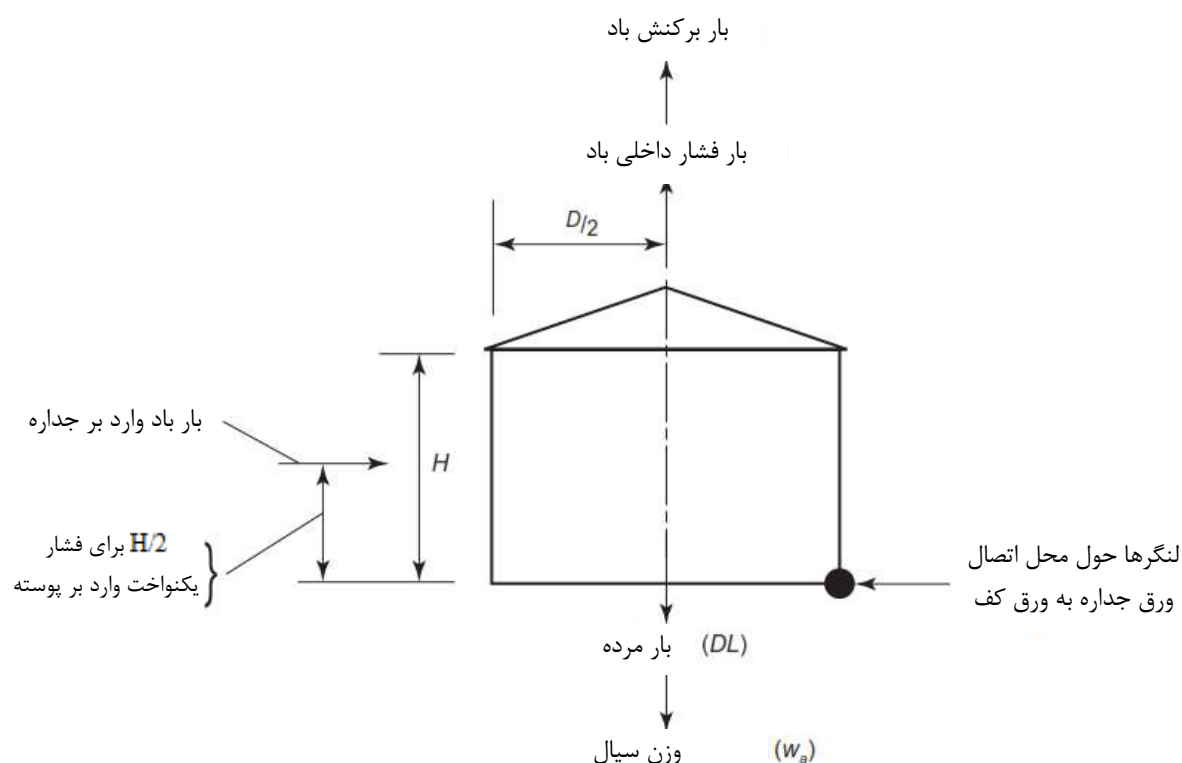
شکل ت-۱- کنترل واژگونی برای مخازن خود مهار
