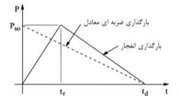
شکل ز-۹- بار فشاری معادل ایده‌آل‌سازی شده [23]
