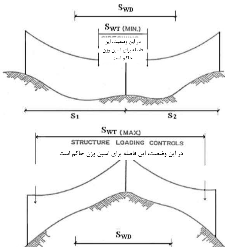
شکل ح-۱- تعریف اسپن باد، S_{WD} و اسپن وزن، S_{WT} حداقل و حداکثر
