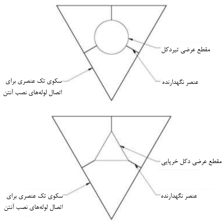
شکل خ-۸- سکوهای کم ارتفاع
