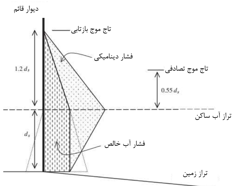
شکل ۳- فشارهای برخورد موج تابشی شکننده قائم روی یک دیوار قائم (تراز آب ساکن یکسان دو سمت دیوار)
