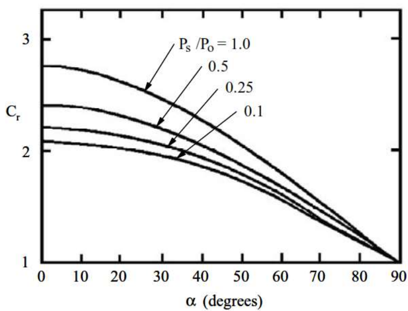
شکل ز-۵- ضرایب بازتاب موج در برابر زاویه برخورد موج فشاری
