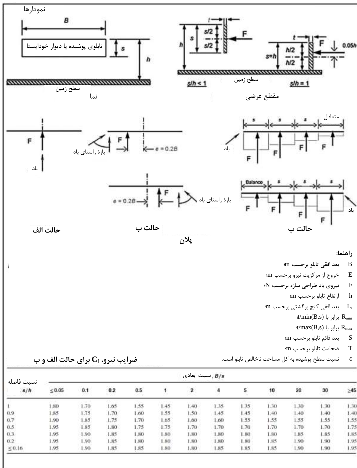
شکل ۲۴- ضرایب نیرو، C_f ، برای دیوارها و تابلوهای پوشیده خودایستا (بدون مهار)- حالت الف و حالت ب
