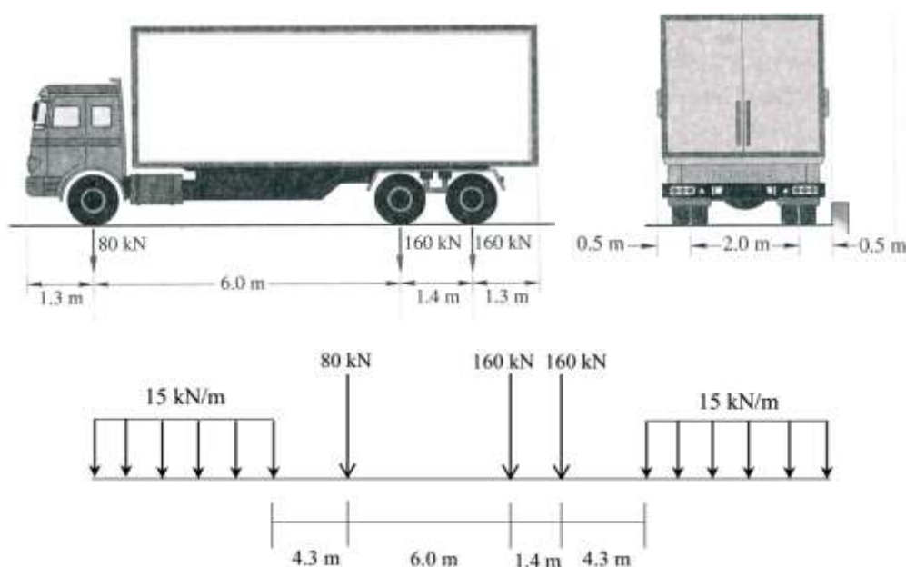
شکل پ-۱- مشخصات بارهای محور ۱ و بار گسترده ۲ در کامیون طراحی (بار زنده عادی) [41]
