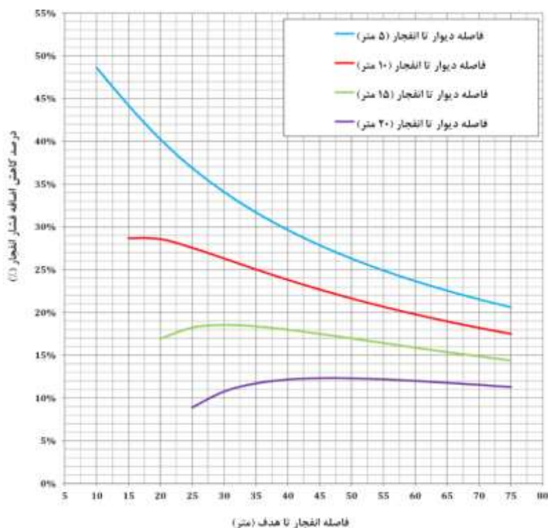
شکل ز-۱۰- نمودار درصد کاهش میزان بار انفجار پشت دیوارهای محافظ
