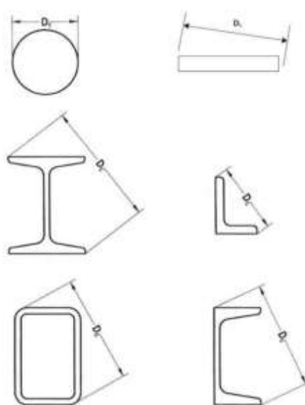
شکل ۲۰- ابعاد مشخصه D_c برای محاسبه مساحت یخ برای انواع مختلف مقاطع
