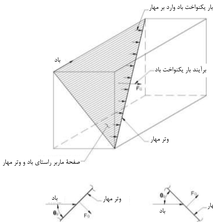
شکل خ-۱۰- نیروی باد وارد بر مهارها
