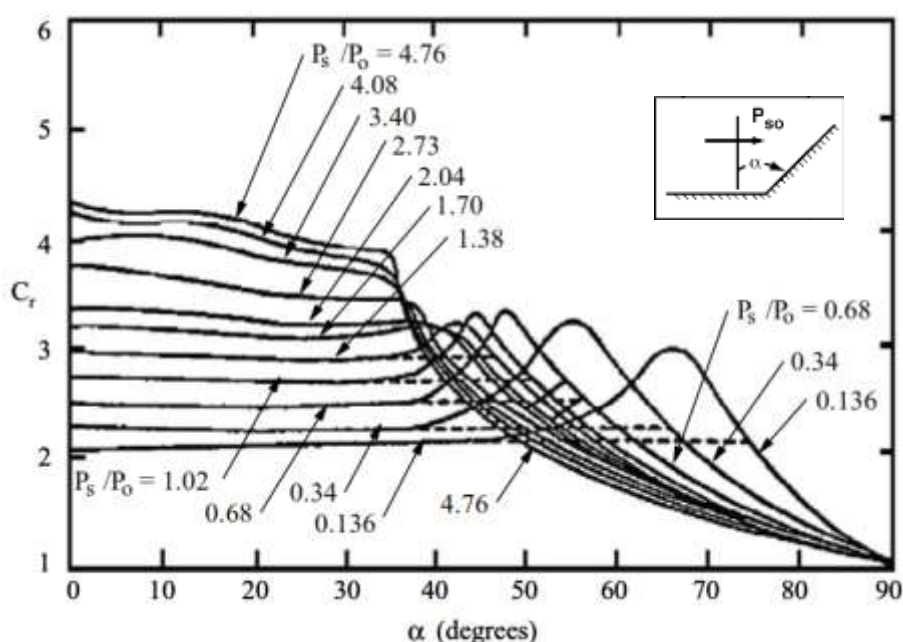
شکل ۴- ضرایب بازتاب موج در برابر زاویه برخورد موج ضربه‌ای
