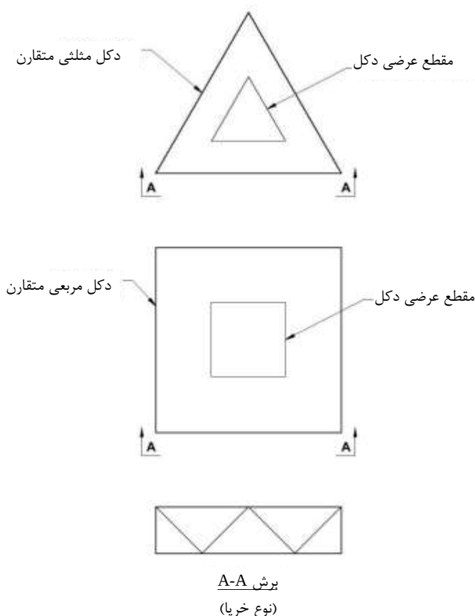
شکل خ-۷- سکوهای قابی یا خریایی متقارن
