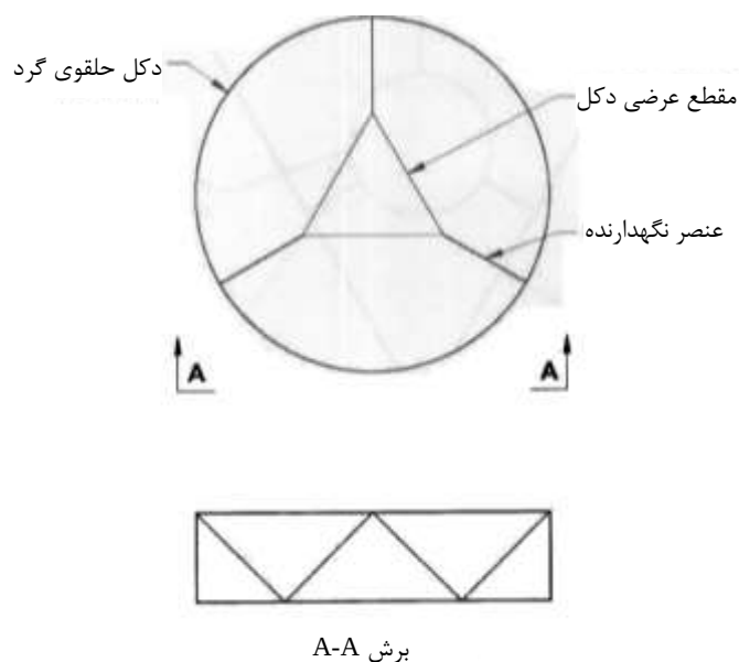
شکل خ-۹- سکوهاى حلقوى گرد
