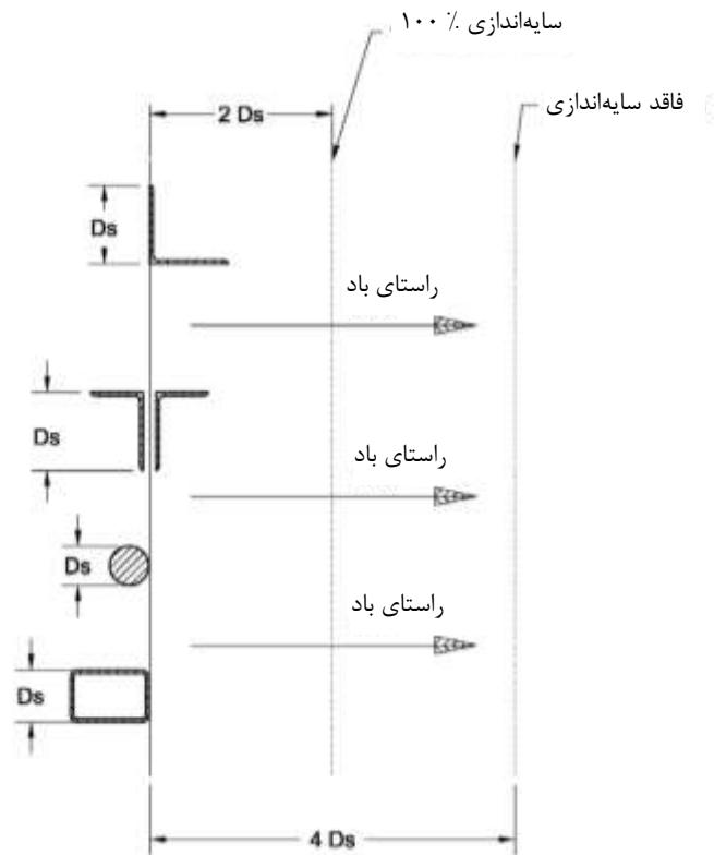
شکل خ-۱۱- محدودیت‌های سایه‌اندازی
