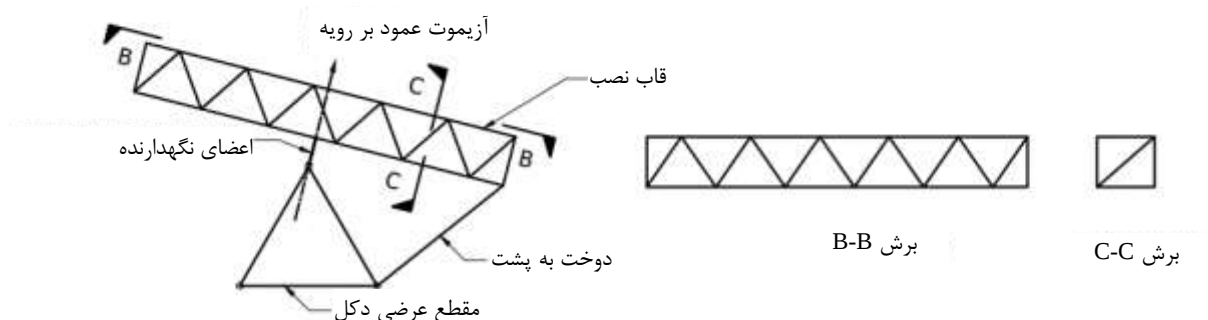
قاب‌های نگهدارنده از نوع خرپایی
