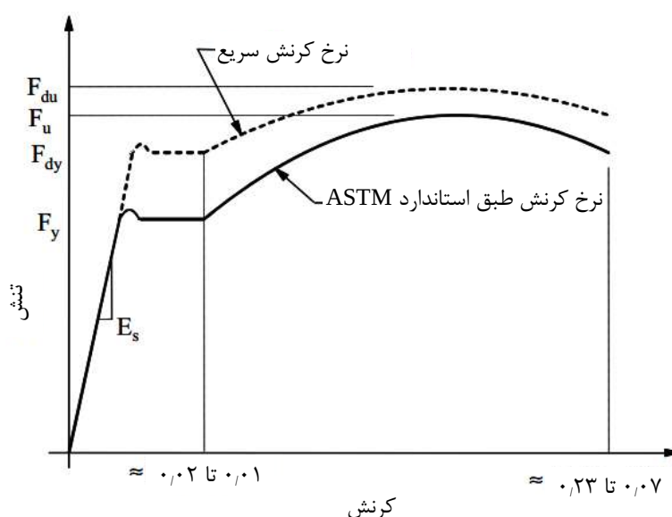
شکل ز-۱۱- اثر نرخ کرنش روی نمودار تنش-کرنش برای فولاد (برگرفته از منبع [24] UFC 3-340-02)
