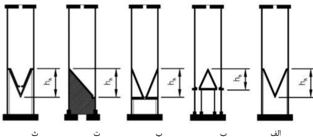
شکل ذ-۱- نمونه‌های از مقاطع عرضی قائم سیلوها به منظور تعیین ارتفاع قیف
