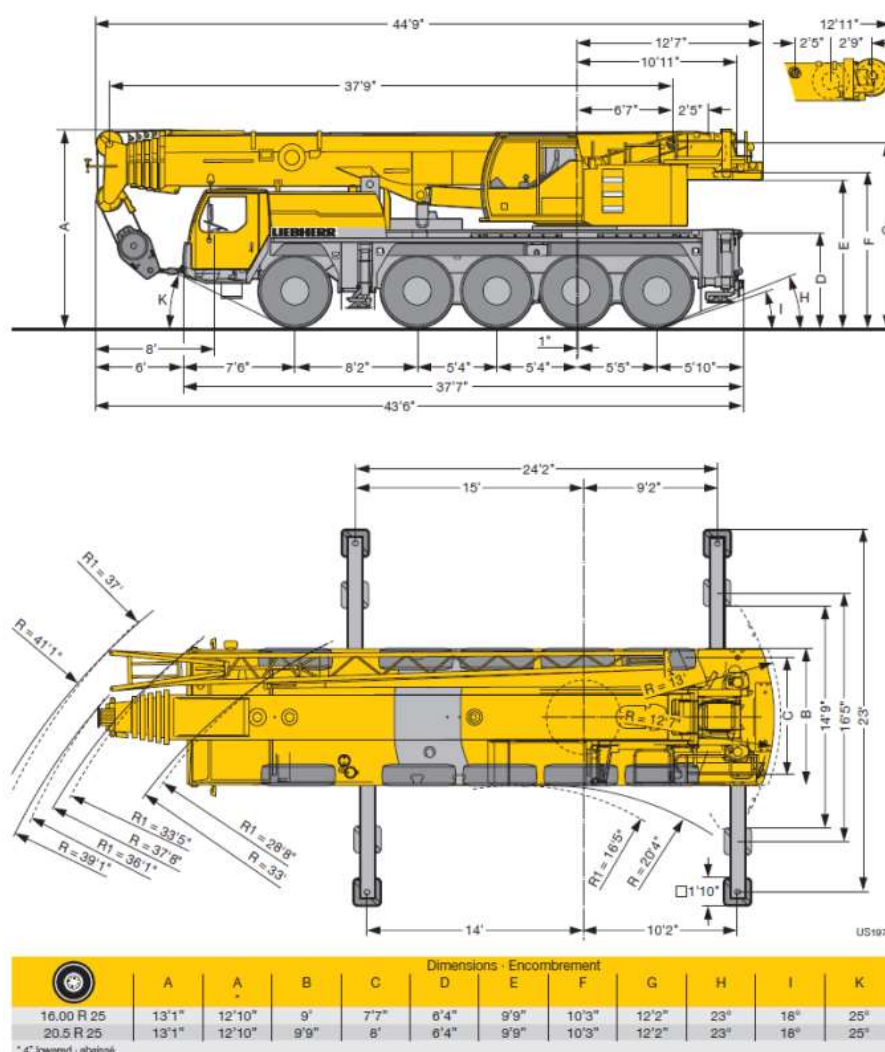
شکل ت-۱- نمونه‌ای از مشخصات هندسی یک جرثقیل متحرک با ظرفیت ۱۰۰ تن
