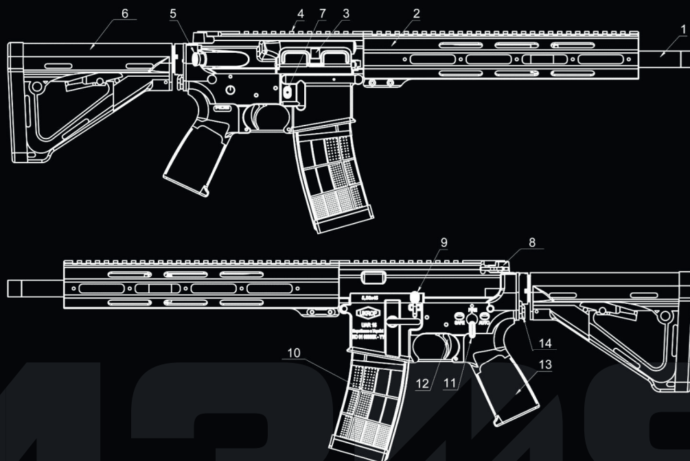
Рис. 3. Органи керування та елементи будови
