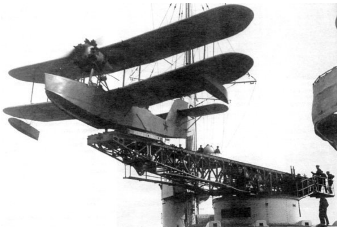
Старт КР-1 с катапульты линкора «Парижская Коммуна»
