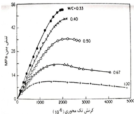
شکل ۱-۶- منحنی تنش- کرنش برای آزمایش فشاری
