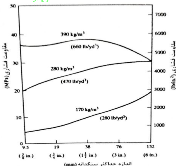
شکل ۶-۷- تاثیر اندازه سنگدانه بر مقاومت فشاری ۲۸ روزه بتن با مقادیر متفاوت سیمان
