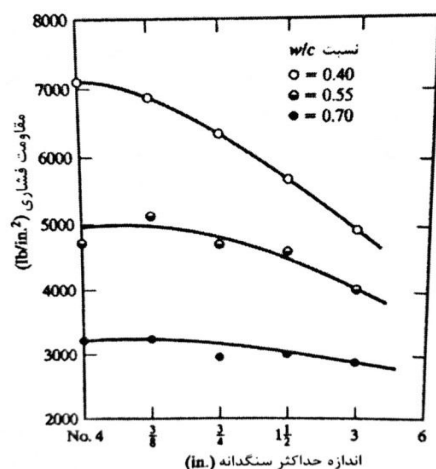
شکل ۵-۷- اندازه حداکثر سنگدانه در مقاومت بتن برای سه نسبت W/C
