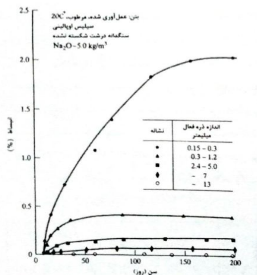
شکل ۸-۱۹- اثر اندازه ذره فعال بر ارتباط بین انبساط و بتن
