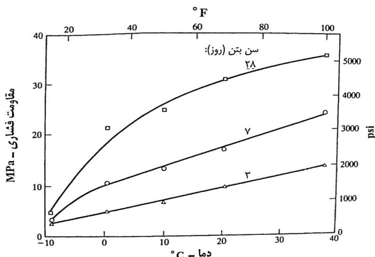
شکل ۶ تاثیر دمای عمل آوری بر مقاومت بتن عمل آوری شده در ۱۰ درجه سلسیوس (۵۰ درجه فارنهایت)
