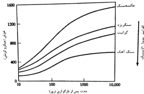
شکل ۶-۶- اثر مدول سنگدانه در خزش
