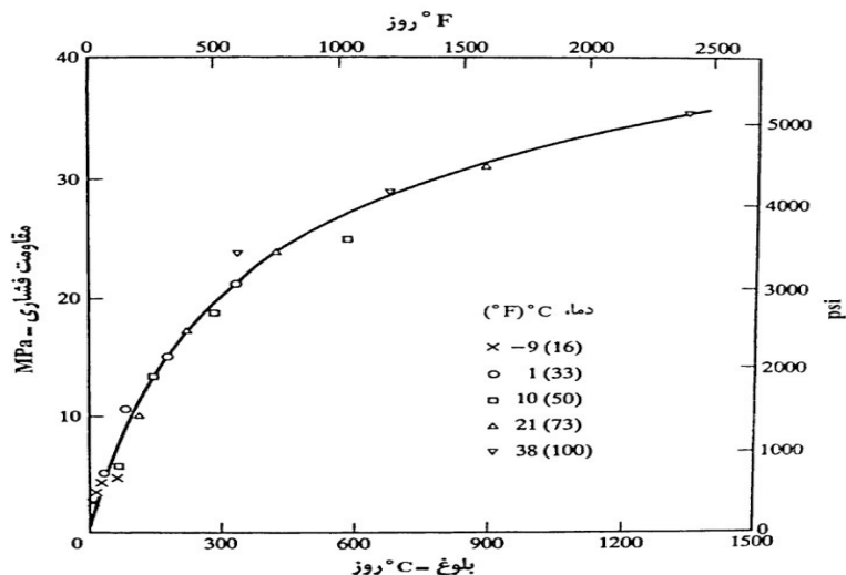
شکل ۷ مقاومت فشاری به عنوان تابعی از بلوغ برای داده های شکل ۶، ۱۰
