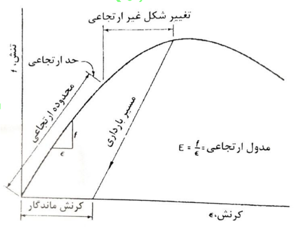
شکل ۲-۶- منحنی تعمیر یافته ی تنش- کرنش برای بتن
