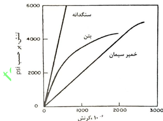
شکل ۷-۱۱- رفتار تنش - کرنش خمیر سیمان، سنگدانه و بتن
