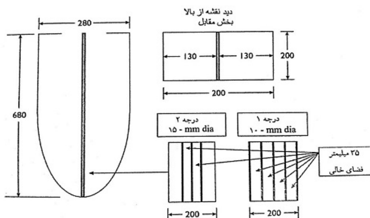
تصویر آزمون جعبه U و موانع (اندازه ها بر حسب میلی متر است)
