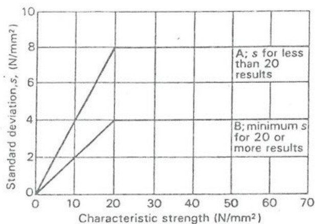
شکل ۱ منحنی های انحراف معیار S
