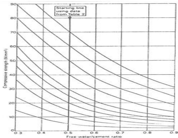
شکل ۳ نمودار نسبت آب به سیمان
