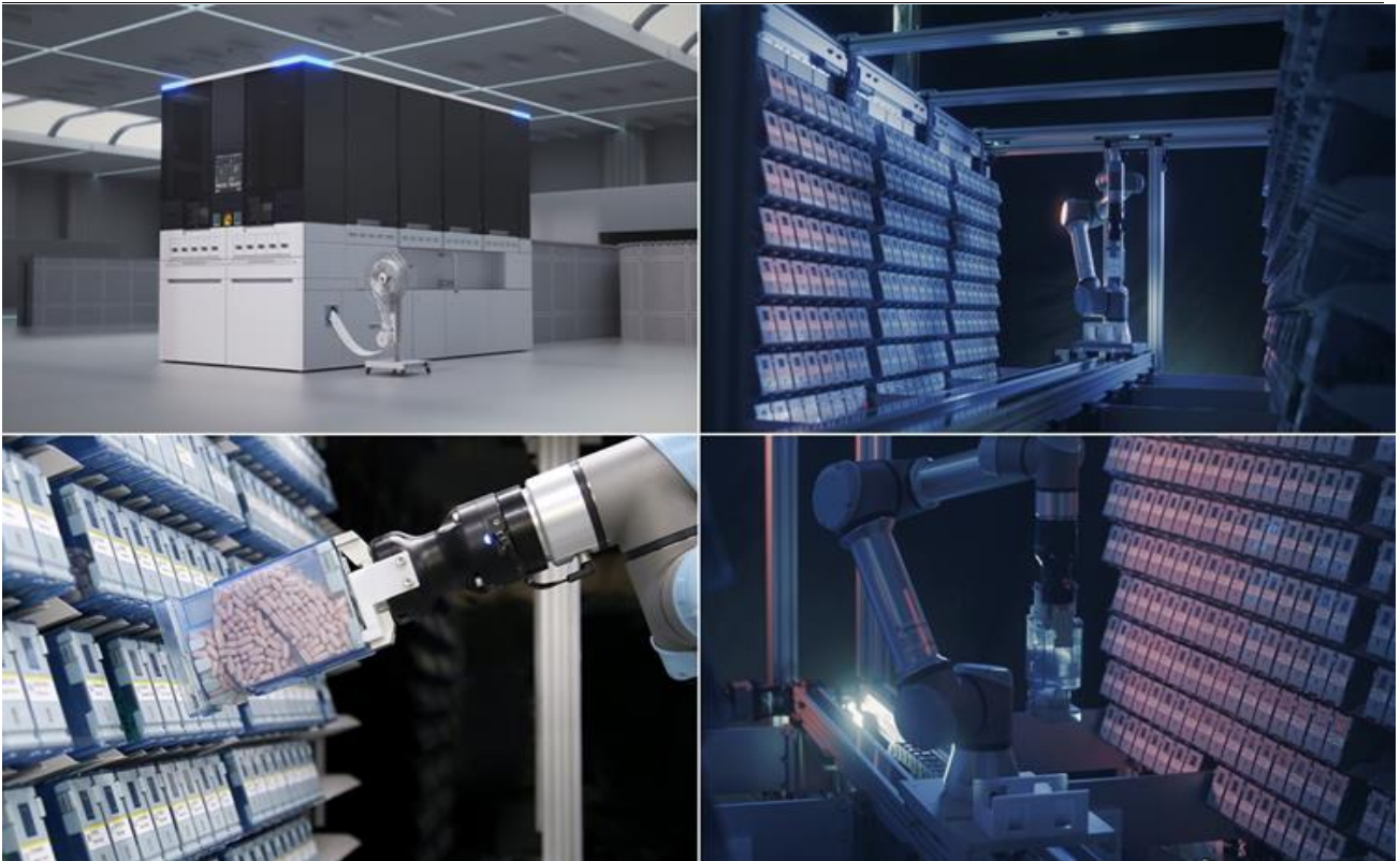
그림9. 제이브이엠의 최첨단 차세대 자동 조제기 MENITH: 다관절 협동 로봇 팔이 이 장비 안에서 캐니스터를 자동으로 교체하고 있다.
