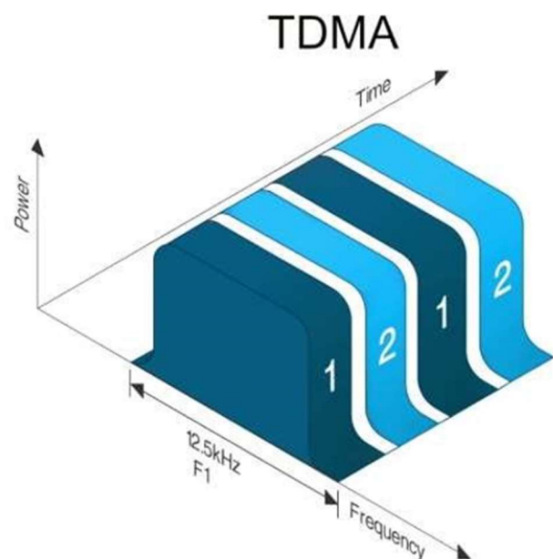
Рис. 32 – Схема работы тайм-слотами на одной частоте
