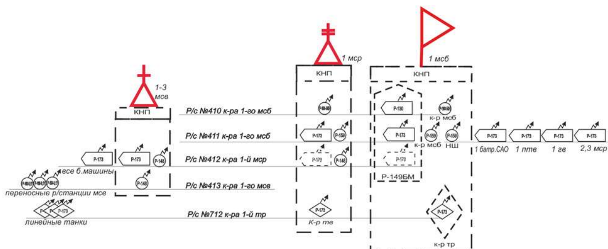
Рисунок 4 – Схема организации радиосвязи в 1-й мср (вариант!) 1
