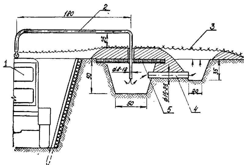
Рис. 4.7. Устройство ямы-глушителя:
