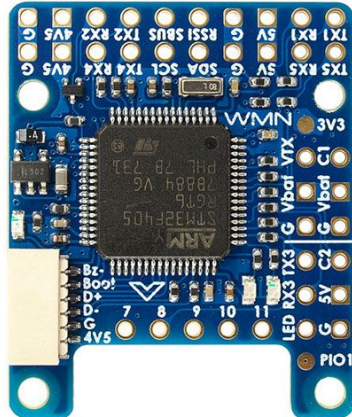
Полётный контроллер Mateksys
