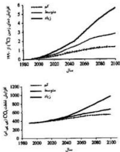
شکل ۳-۲. روند تغییرات افزایش غلظت CO_2 و درجه حرارت تحت سه سناریوی تغییر اقلیم.
