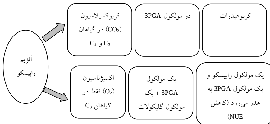
شکل ۳-۳. مسیرهای کربوکسیلاسیون و اکسیژناسیون آنزیم رایبیسکو در مرحله تاریکی فتوسنتز گیاهان C_3 و C_4 .
