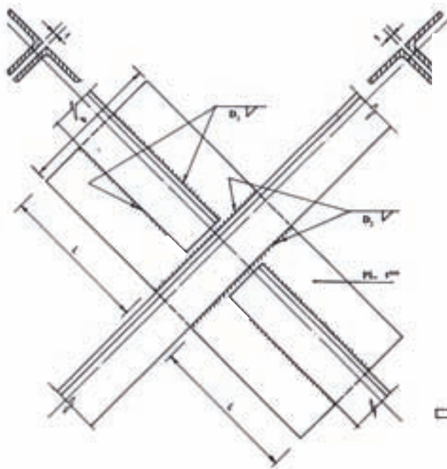
اتصال میانی در بادبند از نیمرخ نبشی زوج
