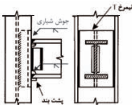
شکل ۸-۱۲- اتصال صلب تیر به جان ستون از نوع
