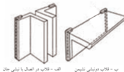
قلاب انتهایی ( برگشت جوش در اتصال ساده)
