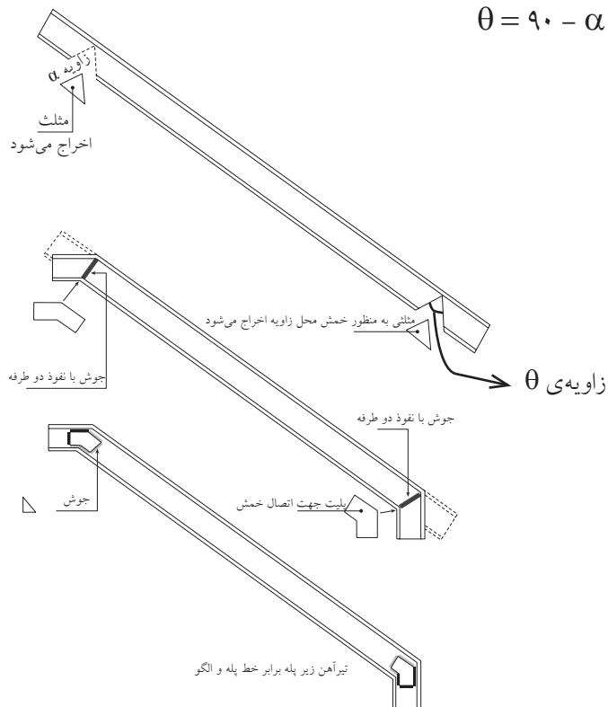
شکل ۸-۳۲- مراحل سه گانه سافت تیر (راه‌پله) (شمشیری)
