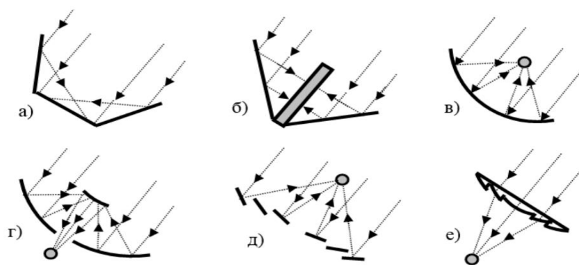
1-rasm. Turli xil konsentratorlarning ko'ndalang kesim sxemalari:
