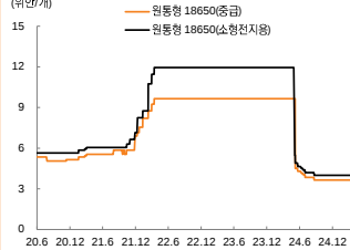
원통형 배터리
