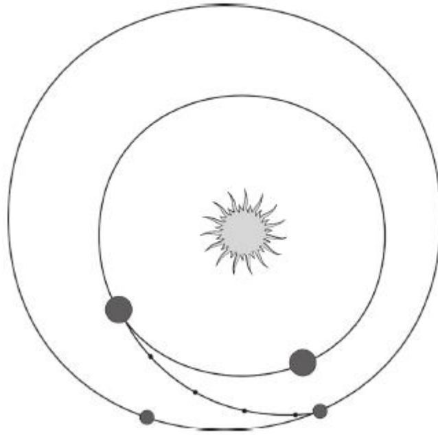
Рис. 7. Переліт до Марса швидкісним ВМК «Голіаф 498»
