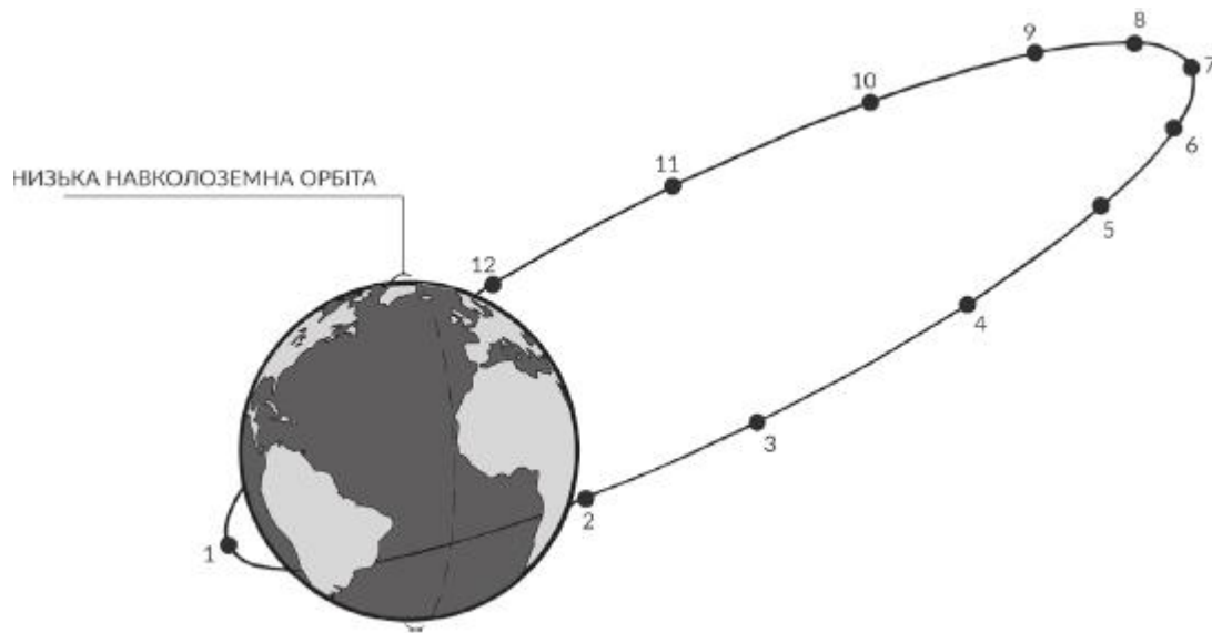
Рис. 5. Висока еліптична навколоземна орбіта
