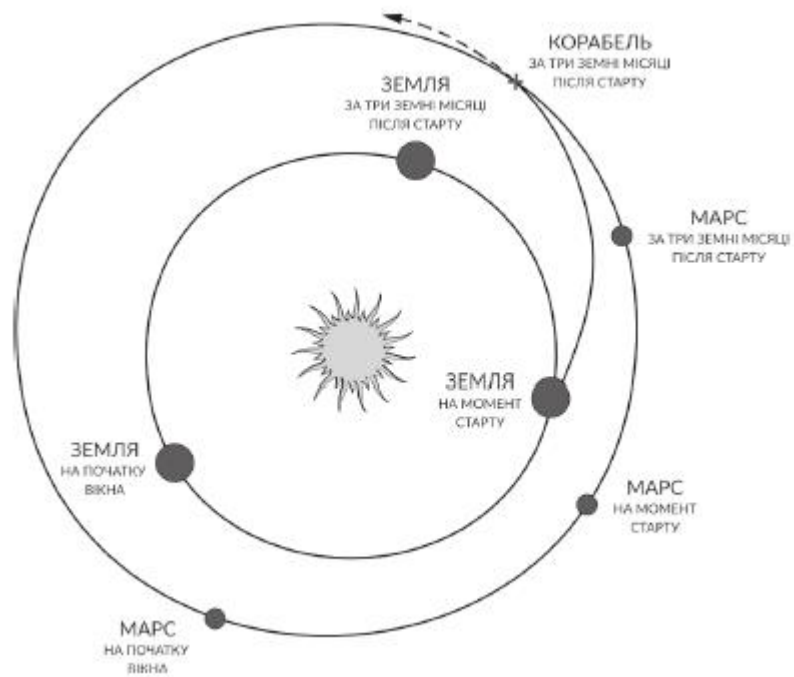
Рис. 8. Неможливість перельоту еліптичною траєкторією після закінчення протистояння
