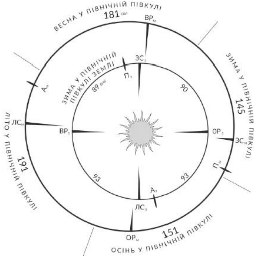
Рис. 2. Конвертація дат із григоріанського у марсіанський календар
