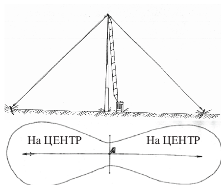
Рис. 101. Диаграмма направленности антенны диполь
