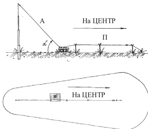
Рис. 100. Диаграмма направленности антенны «Наклонный луч»
