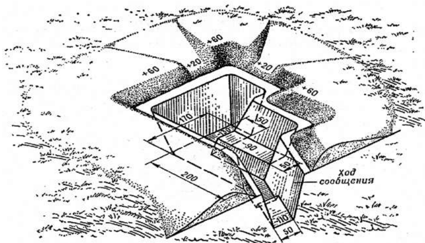
Рис. 139. Открытое сооружение для наблюдательного поста. На устройство сооружения с помощью пехотной лопаты требуется 7,5 чел.-ч, а с помощью саперной лопаты — 5 чел.-ч
