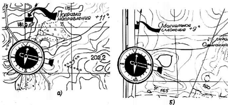
Рис. 118. Ориентирование карты по компасу:
