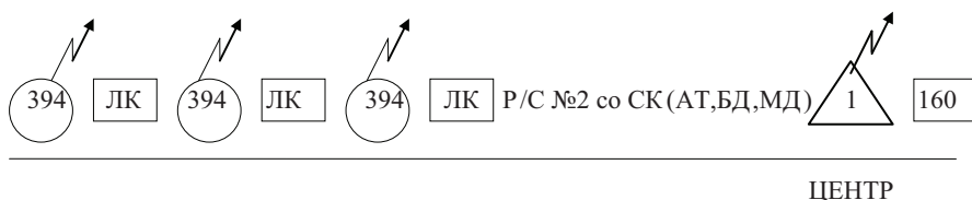
Рис. 98. Схема организации радиосети (вариант)
