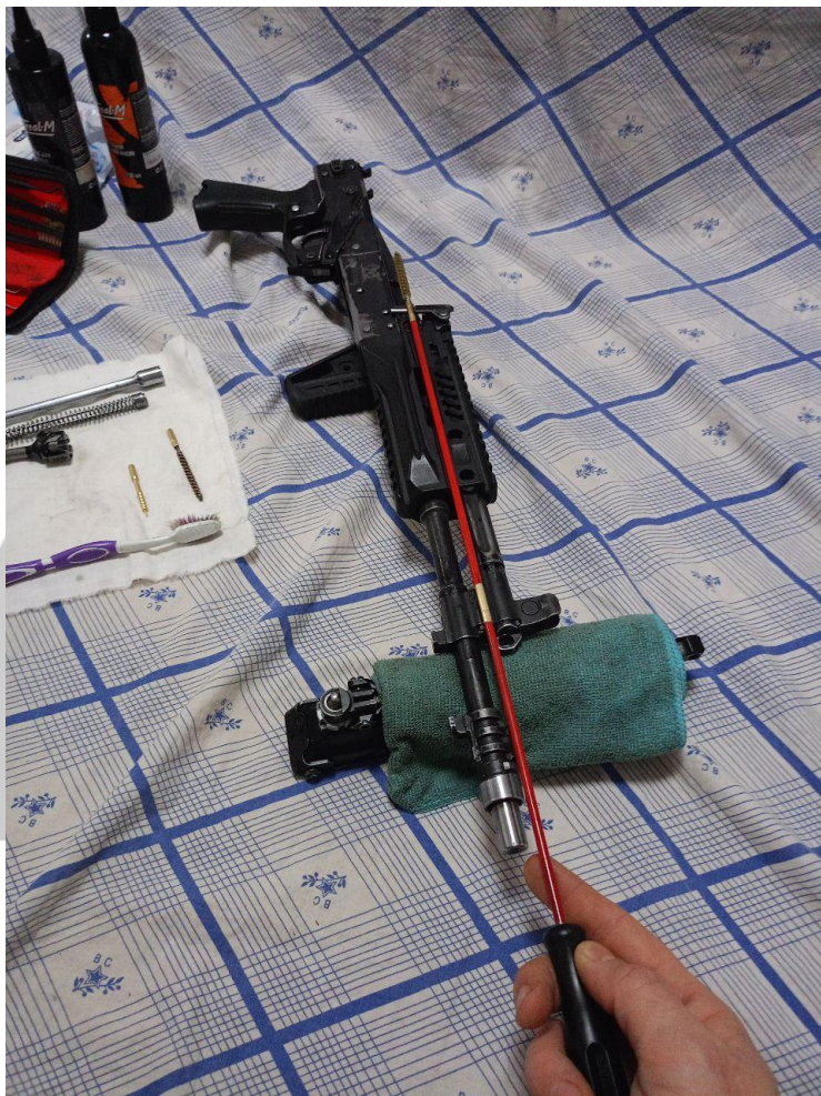
Рисунок 36. Соотношение длины двух колен шомпола и длины ствола АК-12
