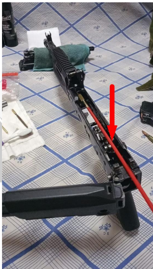
Рисунок 38. Процесс заведения шомпола с ершом в канал ствола
