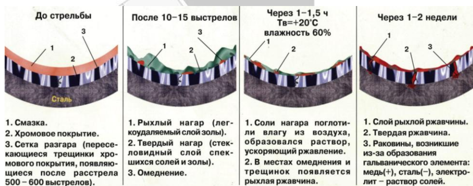
Рисунок 1. Процесс коррозии внутренней поверхности ствола
